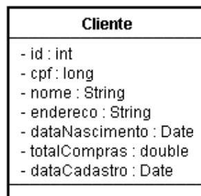
Figura 7 - Classe Cliente
